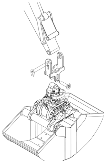
Grappin avec suspension supérieure par noix de cardan
