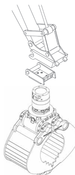
Grappin avec platine vissée pour système d'attache rapide
