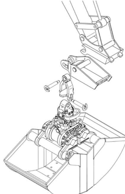
Grappin avec suspension supérieure par noix de cardan et système d'attache rapide
