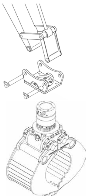
Grappin avec platine fixe
